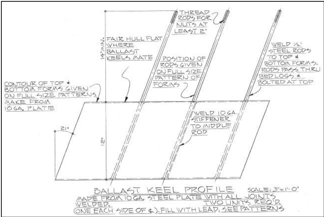
Glen-L 25 PW ballast keel detail
